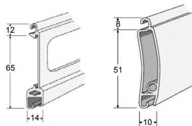
Lamellprofil GR 6502 och VST 5110
